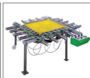
Siebspanngeräte
